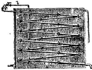
Рис. 4. Холодильникъ для сгущенія продуктовъ перегонки Д.
