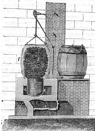
Рис. 11. Возгонка нафтalina.
