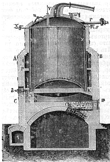
Рис. 1. Вертикальный разрѣзъ котла для перегонки дегтя по линіи Еф .
