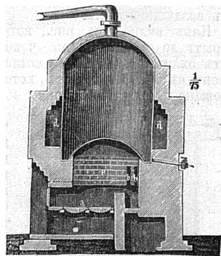
Рис. 6. Типъ англійскаго котла для перегонки дегтя.
