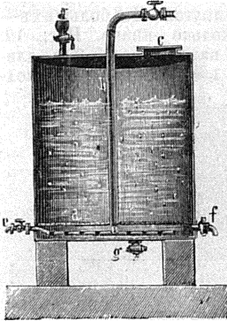
Рис. 10. Другой типъ мѣшалки для химической обработки продуктовъ перегонки изъ Д.
