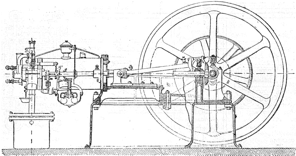
Рис. 3. Двигатель Отто.
