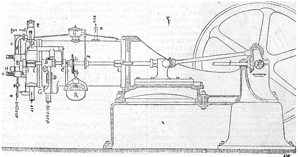
Рис. 2. Двигатель Отто.
