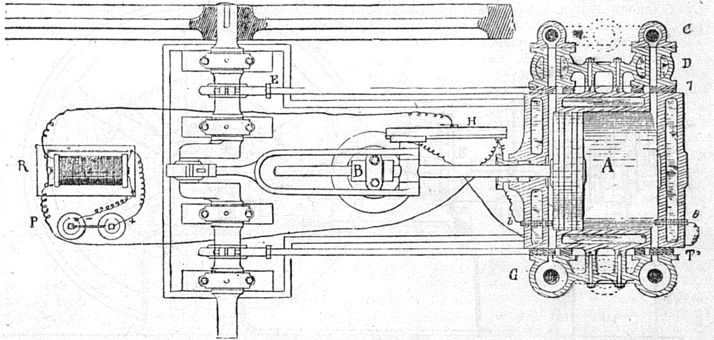
Рис. 1. Двигатель Ленуара.
