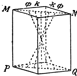
Черт. 1. Схематическое изображение двуосного кристалла; \kappa < \varphi . MNPQ —положеніе плоскости оптических осей.
