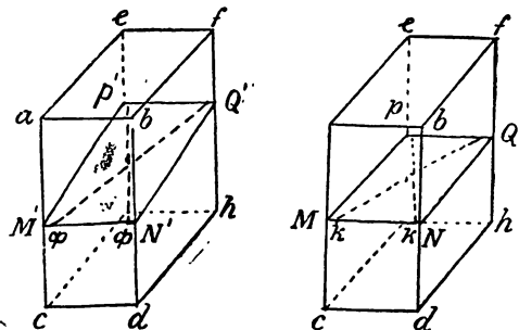
Черт. 11. Ортоклазъ (маленькій полевой шпатъ). M N Q P — положеніе плоскости оптическихъ осей для лучей краснаго цвѣта. M' N' Q' P' — положеніе плоскости оптическихъ осей для лучей фиолетоваго цвѣта ( \kappa > \phi ). Плоскость оптическихъ осей измѣняетъ при этомъ свое положеніе, поворачиваясь около линіи параллельной ребру кристалла ab .
