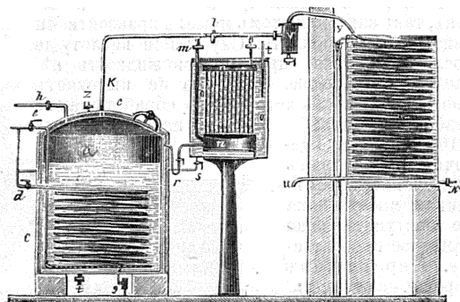
Рис. 9. Дефлегмаціонный аппаратъ.
