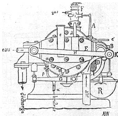
Рис. 4. Двигатель Отто.
