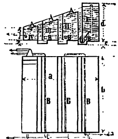
Рис. 5. Приборъ для удаленія воды изъ дегтя.
