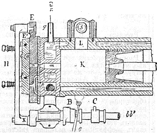
Рис. 5. Золотникъ и поршень D . Отто.
