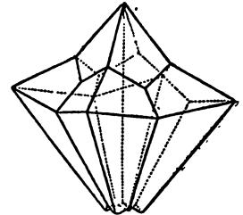
Фиг. 5. Мѣдный колчеданъ.
