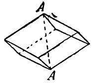
Черт. 10. Кальцитъ (отрицательный).
