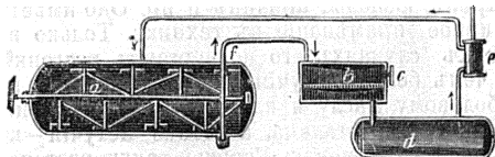
Рис. 15. Приборъ для очистки антрацена экстрагированіемъ примѣсей.
