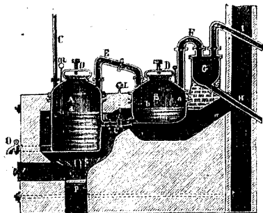
Рис. 7. Приборъ для непрерывной перегонки дегтя.
