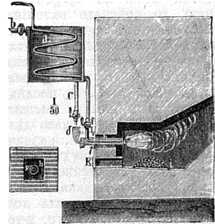
Рис. 14. Приспособленіе для сжиганія тяжелого каменноугольного масла въ топкахъ паровыхъ котловъ и пр.
