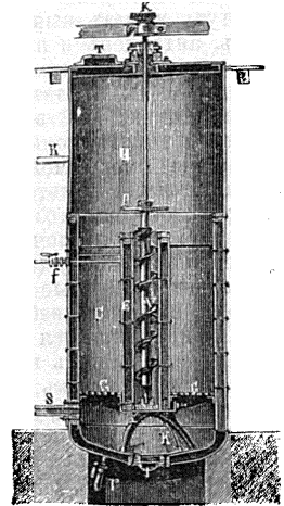
Рис. 16. Мѣшалка для приготовления смолъ разныхъ качествъ
